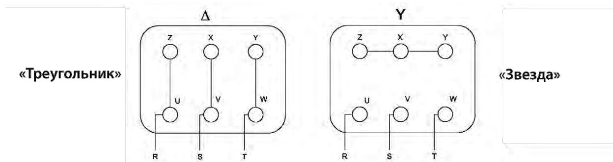
Схемы подключения: «треугольник» и «звезда»
